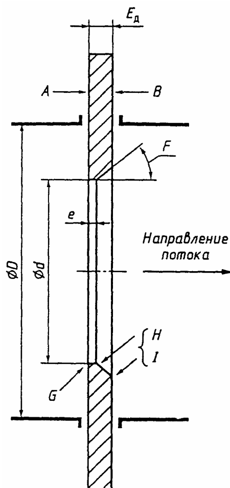
Рисунок 3 - Стандартная диафрагма
