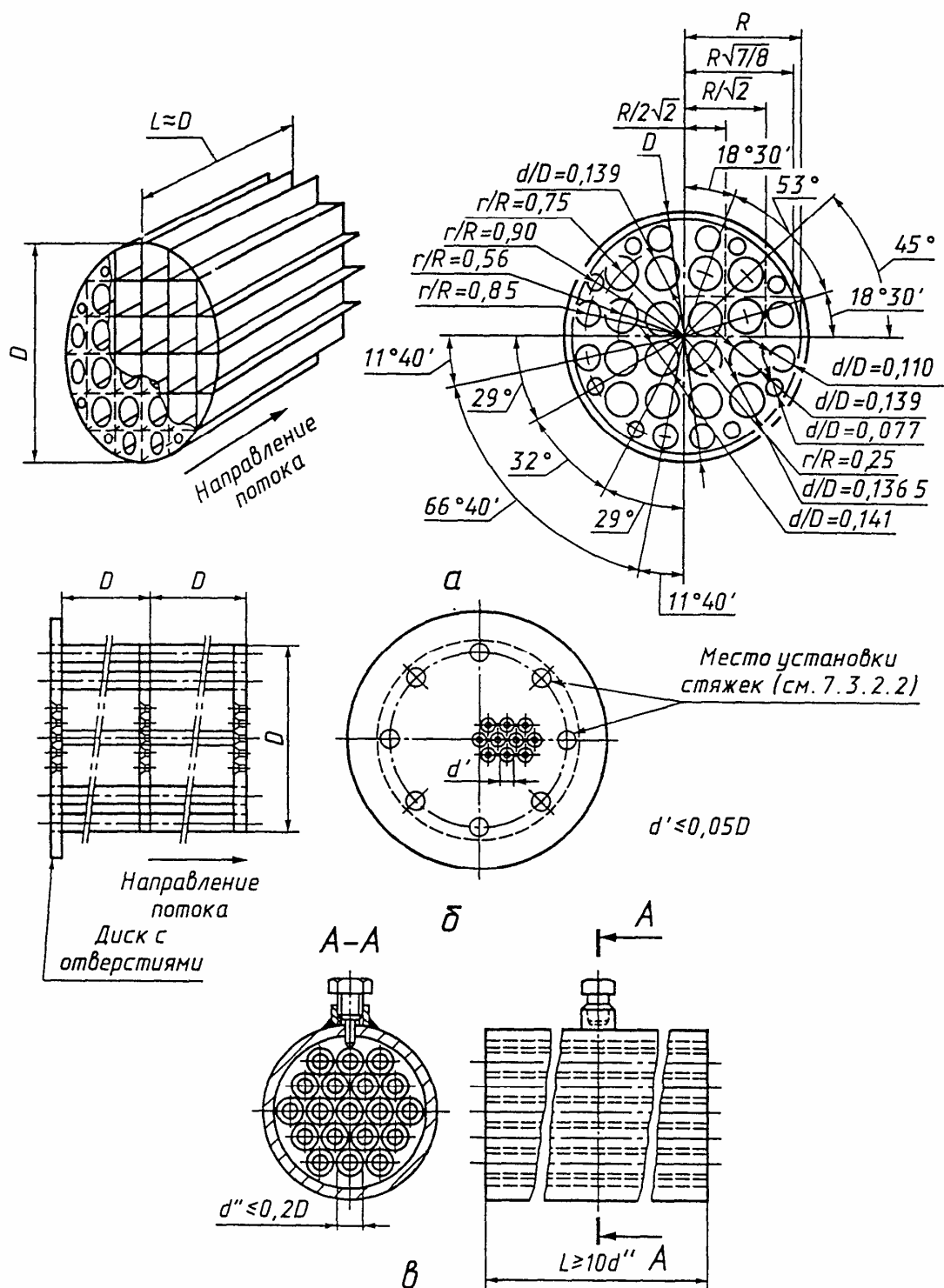
Рисунок 1 – Струевыпрямители
