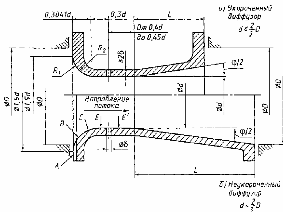
Рисунок 9 - Сопло Вентури
