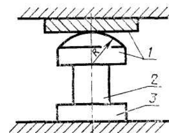
1 и 3 — опоры; 2 — образец
