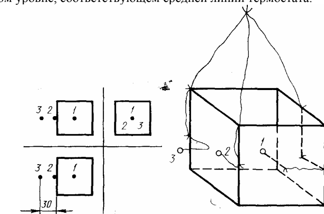
1,2,3 — рабочие спай термоэлектрических преобразователей
