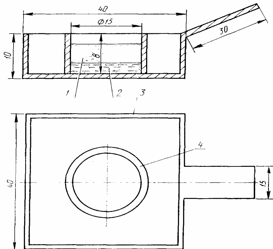
1 — песок; 2 — жидкость; 3 — лодочка; 4 — цилиндрическая емкость Черт. 24
